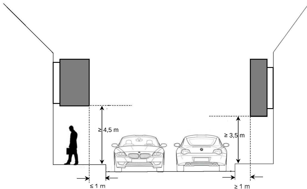
Figure 1 Installation des supports publicitaires, sauf dans le « shared space »
