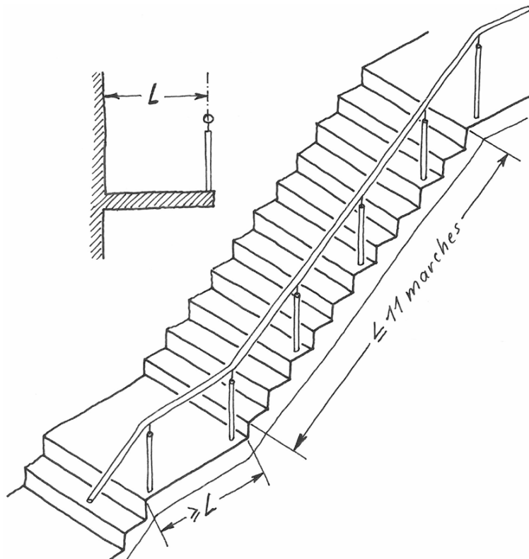
Figure 13 Géométrie d'un escalier
