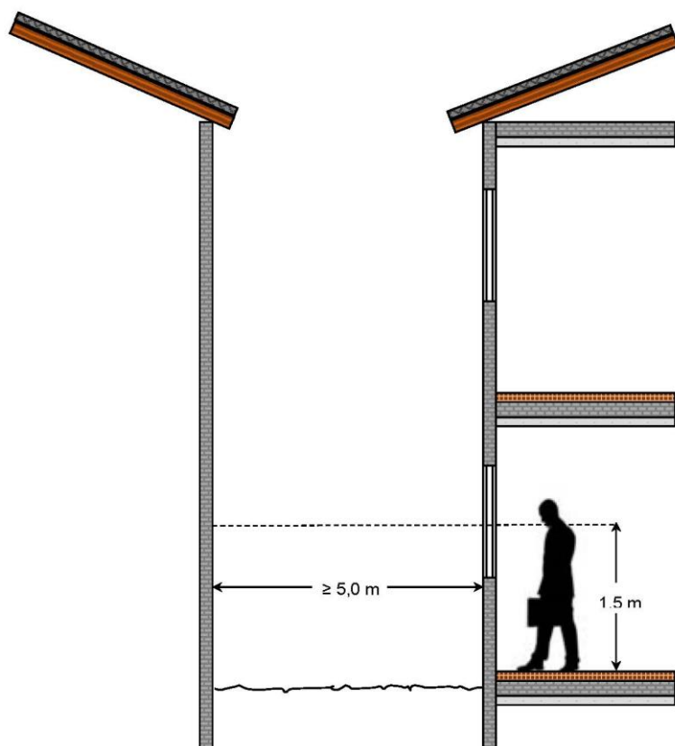
Figure 9 Vues directes et horizontales depuis les pièces destinées au séjour prolongé de personnes vers l'extérieur
