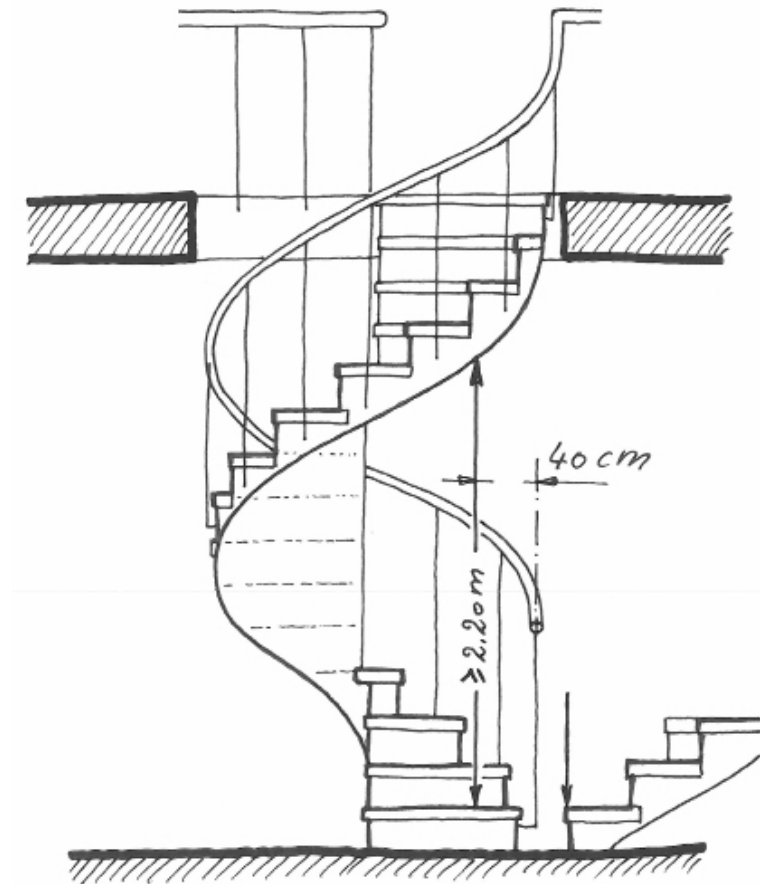
Figure 14 Géométrie d'un escalier en colimaçon ou à marches tournantes
