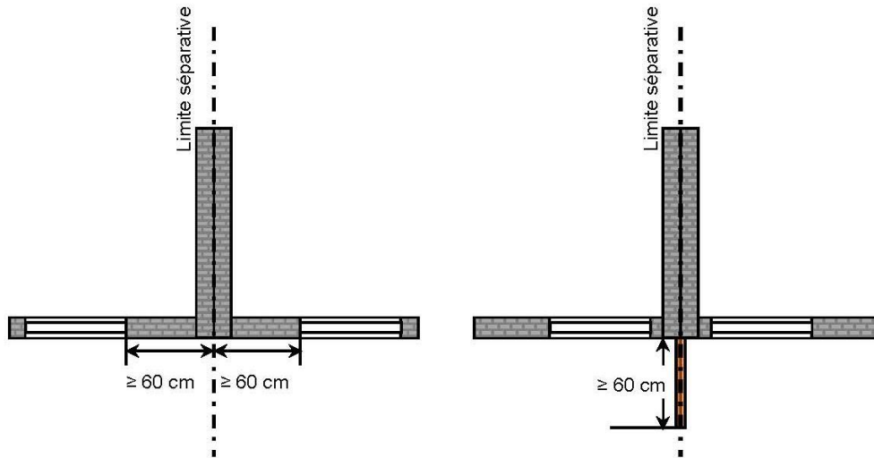
Figure 11 Distance entre ouvertures
