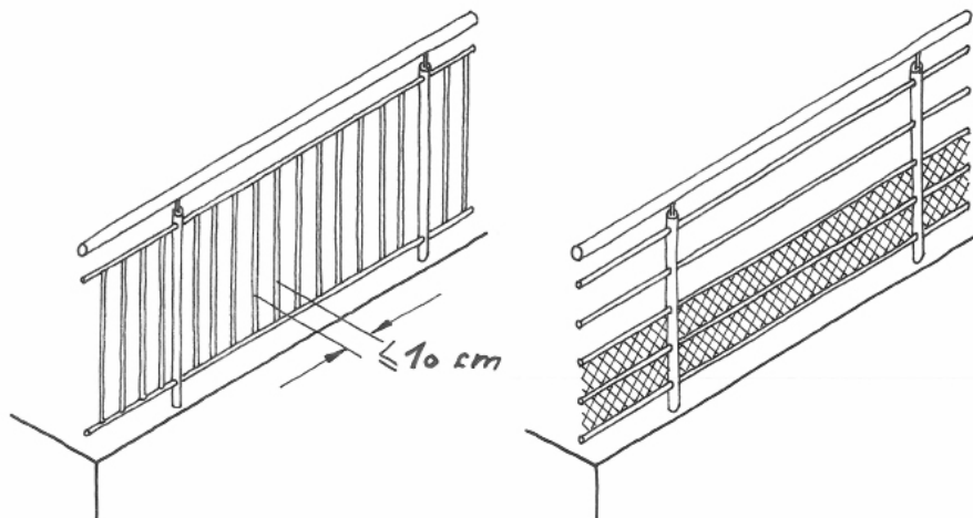
Figure 16 Géométrie des garde-corps (entraxe entre barreaux verticaux et dispositif empêchant d'y grimper)
