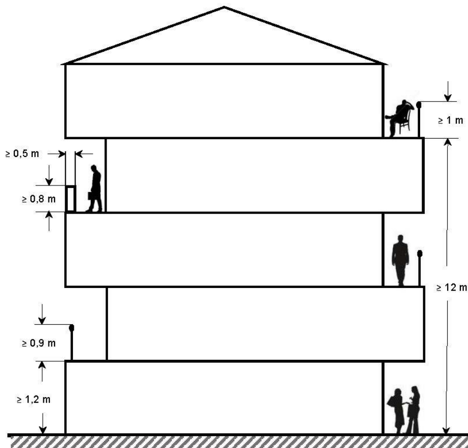
Figure 15 Hauteur des garde-corps
