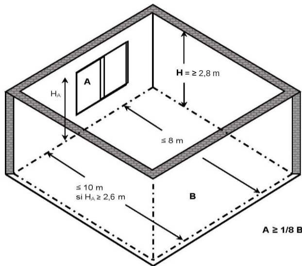
Figure 12 Distance entre le point le plus éloigné à la source lumineuse naturelle et cette source lumineuse
