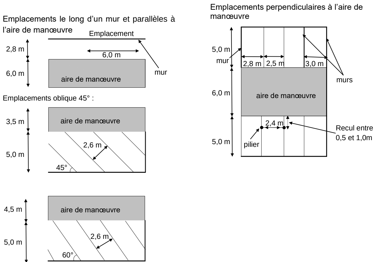
Figure 7 Dimensionnement des emplacements pour voitures
