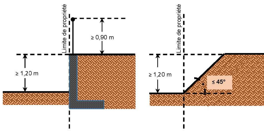
Figure 5 Clôtures et aménagements en bordure des limites séparatives
