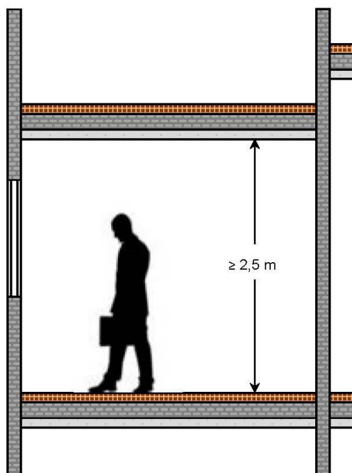
Figure 8 Hauteur libre sous plafond dans les pièces destinées au séjour prolongé de personnes
