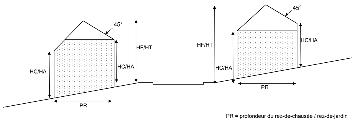
Gabarit type dans un terrain en pente >15%
